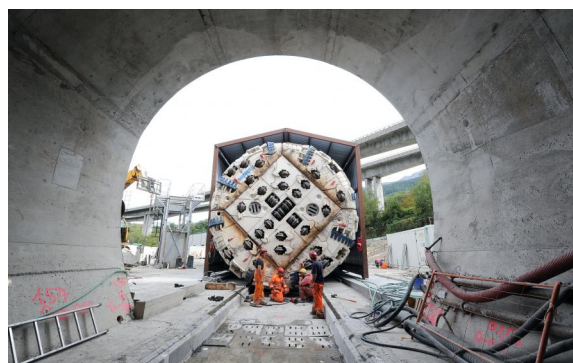
Chantier de la Maddalena - Italie
