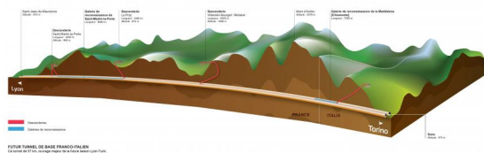
Futur tunnel de base du Lyon-Turin, long de 57,5 km
